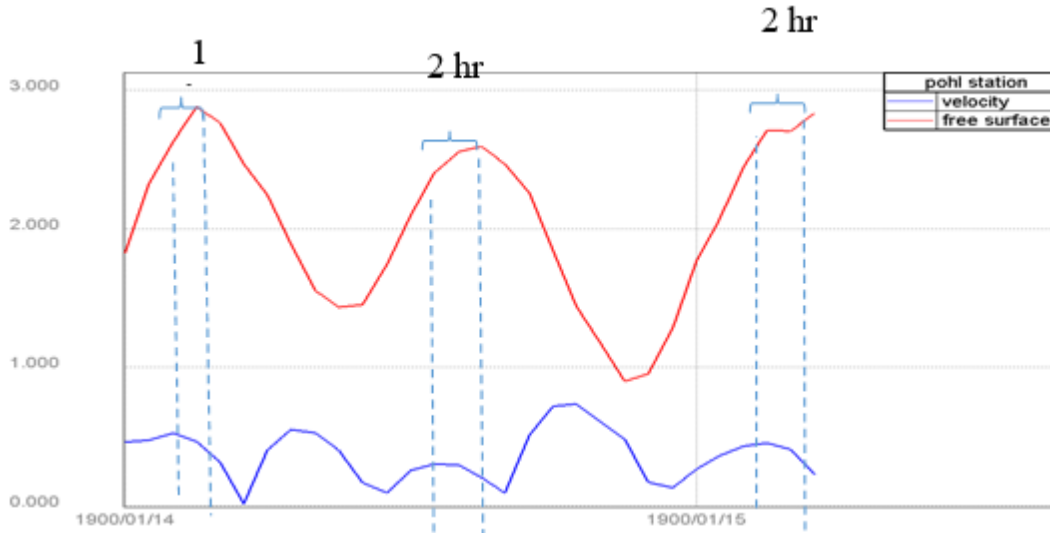
شکل ۹- تراز آب (متر) و سرعت (متر بر ثانیه) برای ۲۹ ساعت در ایستگاه پل
