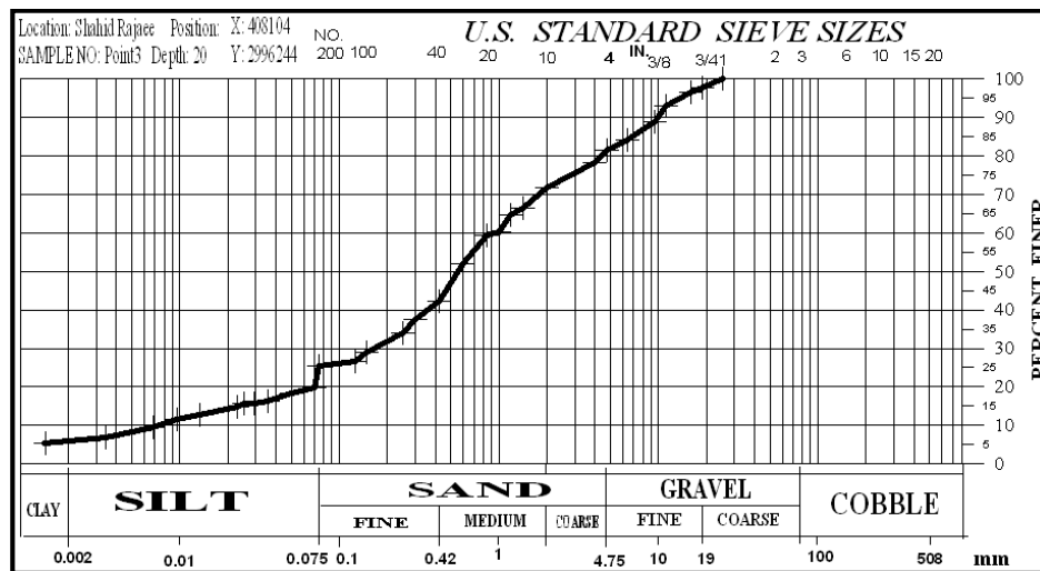
شکل ۵- نتایج دانه بندی در سه ایستگاه کانال دسترسی بندر شهید رجایی
