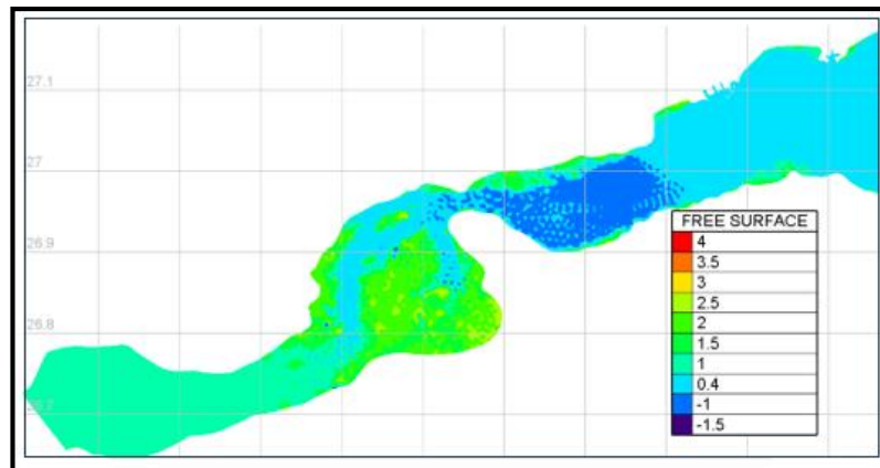
شکل ۶- تراز سطح آب مدل شده Fig. 6- Simulated water level
